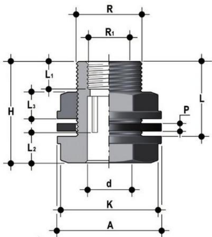
Танк-адаптер ПВХ FIP 25x1 1/4x1
