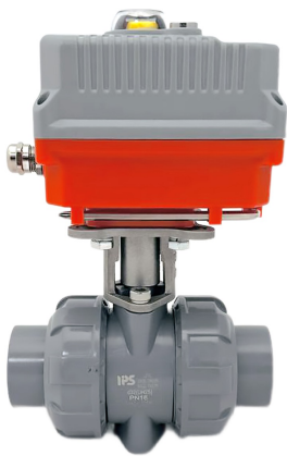
Шаровой кран IVKD ХПВХ с эл.приводом (площадка IPQ) 220V, муфтовые окончания d32 (DN25)
