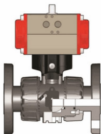
Шаровой кран VKD ПВХ с пневмоприводом НЗ с фланцевыми окончаниями, EPDM, FIP d50 (DN40)
