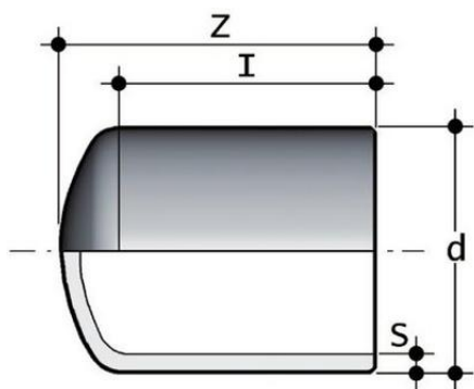
Заглушка для стыковой сварки PP-H FIP (PN10) d140 SDR11 PN10
