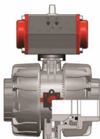
Шаровой кран VKD ПВХ с пневмоприводом ДвД с муфтовыми окончаниями, EPDM, FIP d110 (DN90)
