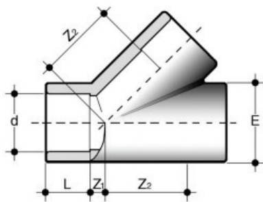
Тройник равнопроходной клеевой 45° ПВХ FIP d32
