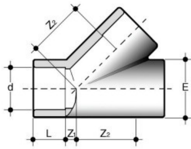
Тройник равнопроходной клеевой 45° ПВХ FIP d160
