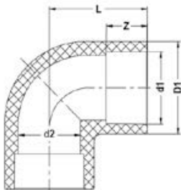
Отвод для раструбной сварки 90° PP-H IPS d63 PN10
