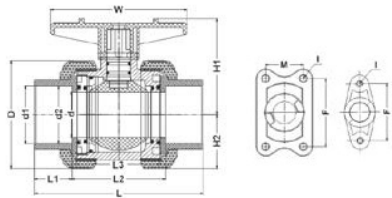
Кран шаровый ХПВХ муфтовый промышленный EPDM IPS d63 (DN50)
