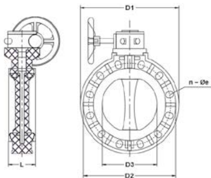
Дисковый затвор IFK ПВДФ с редуктором d8" (DN200)
