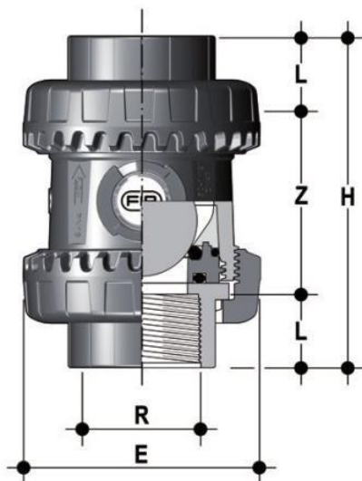
Шаровой обратный клапан SXEFV ПВХ; с резьбовыми окончаниям, FKM, FIP R1¼" (DN32)
