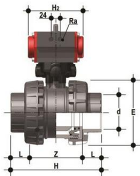
Шаровой кран общего применения VXE ХПВХ с пневмоприводом двойного действия ДвД с муфтовыми окончаниями d90 (DN80)
