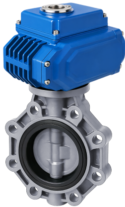
Дисковый затвор IFK ХПВХ с электрическим приводом 220V AC, FKM, IPS d110 (DN90)
