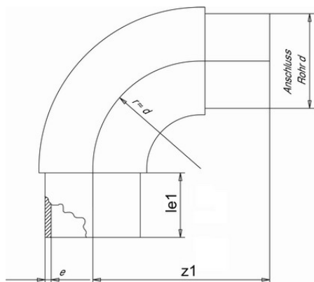
Изгиб 90° PP-H Simona d315 SDR11 PN6
