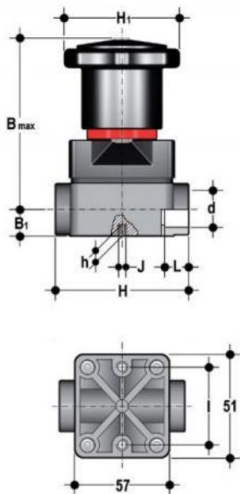
Компактный мембранный клапан CM ПВДФ с муфтовыми окончаниями d20 (DN15)
