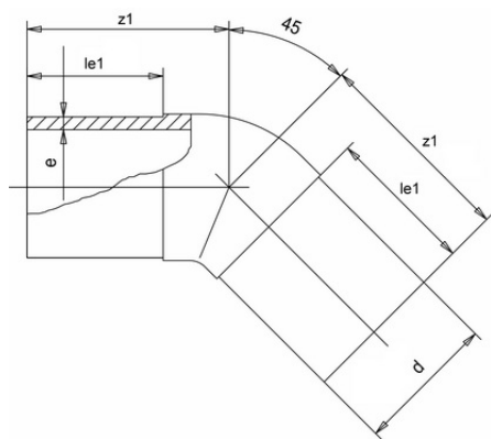
Отвод ПВДФ 45° (Simona) d140 SDR33 PN10
