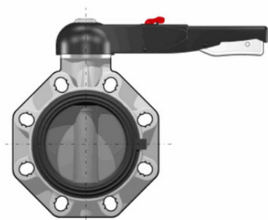
Дисковый затвор ПВХ FKOVL с рукояткой, EPDM, FIP d63 (DN50)
