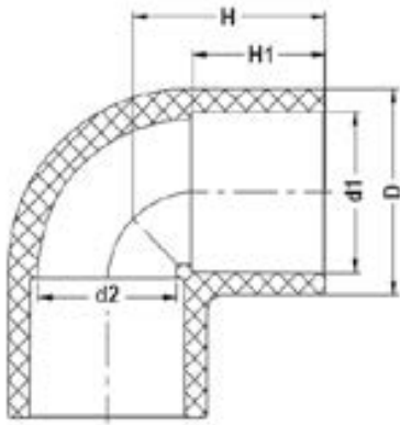
Отвод ПВДФ 90° (IPS) d110 PN 16
