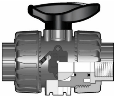
Шаровой кран промышленного применения VKD с резьбовыми окончаниями (уплотнение EPDM) PP-H R2" (DN50)
