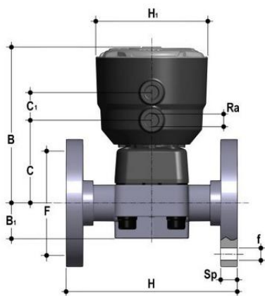
Мембранный клапан DK с пневмоприводом H3, PN6 с фланцевыми окончаниями (уплотнение EPDM/мембрана EPDM) PP-H d32 (DN25)
