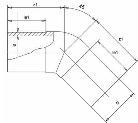
Отвод ПВДФ 45° (Simona) d75 SDR21 PN16
