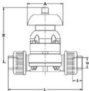
Мембранный клапан IDK PBX с муфтовыми окончаниями, PTFE, IPS d75 (DN65)
