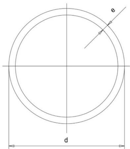
Напорная труба РР-Н Симона, PN4 d1000
