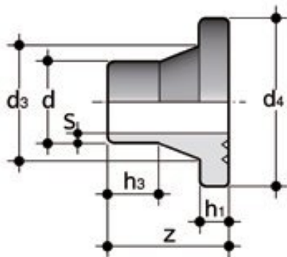
Бурт под фланец для стыковой сварки PP-H FIP d200 SDR17.6 PN6
