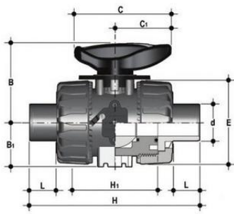
Шаровой кран ПВХ для регулирования потока VKR со втулочными окончаниями, FKM, FIP d40 (DN32)
