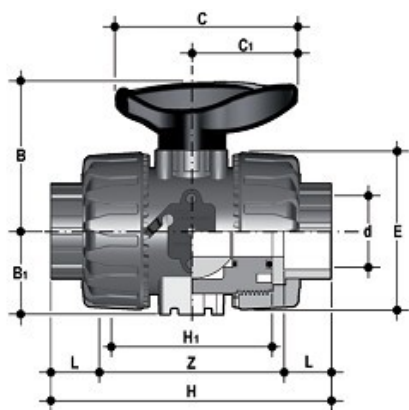
Шаровой кран ПВХ промышленного применения VKD/SHX с муфтовыми окончаниями, EPDM, FIP d40 (DN32)
