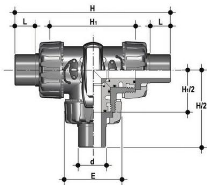
3-х ходовой шаровой кран ПВХ ТКД с втулочными окончаниями, Т-шар, FKM, FIP d20 (DN15)
