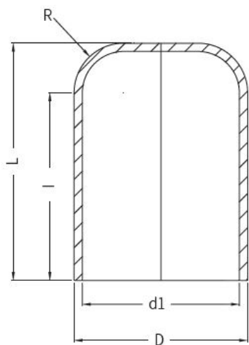
Заглушка ПВДФ для стыковой сварки d32 PN 16
