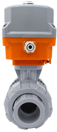
Шаровой кран IVKD ХПВХ с эл.приводом 24V DC, муфтовые окончания d90 (DN80)
