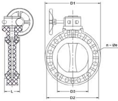
Дисковый затвор IFK ПВДФ с редуктором d10" (DN250)
