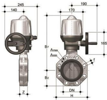
Дисковый затвор FK ПВДФ с эл.приводом 24V AC/DC d14" (DN350)
