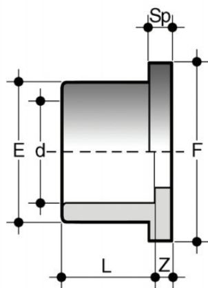
Бурт под фланец ПВХ FIP d90
