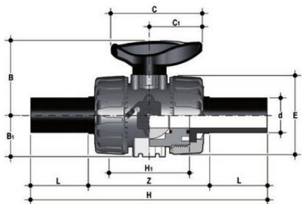
Шаровой кран промышленного применения VKD с патрубками из ПЭ (CVDE) (уплотнение FKM) PP-H d25
