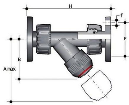
Грязевой фильтр RVUOM с фланцевыми окончаниями (уплотнение EPDM) PP-H d32 (DN25)
