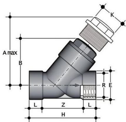
Угловой обратный клапан VRFV ПВХ с резьбовыми окончаниями, EPDM, FIP R3" (DN80)
