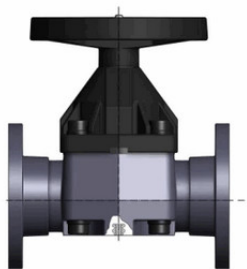
Мембранный клапан VMOM с фланцевыми окончаниями (уплотнение FKM / мембрана FKM) PP-H d90 (DN80)
