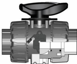
Шаровой кран ПВХ для регулирования потока VKR с муфтовыми окончаниями, EPDM, FIP d40 (DN32)
