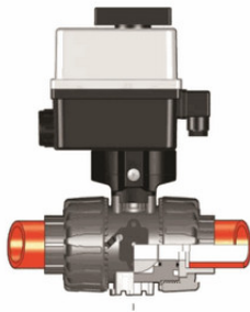
Шаровой кран VKD ПВДФ с эл.приводом 90-240V, муфтовые окончания d20 (DN15)
