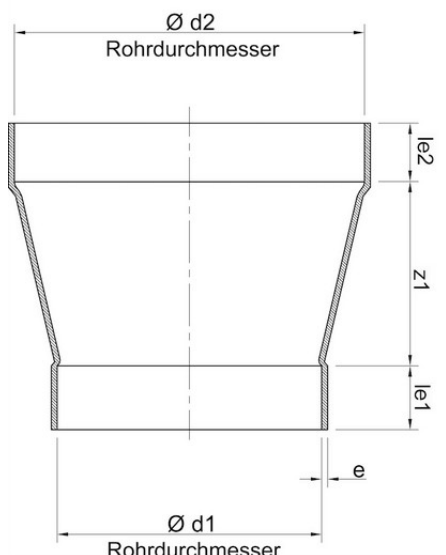
Муфта переходная PPs 630x450
