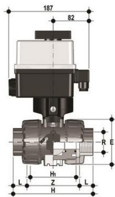
Шаровой кран VKD ПВХ с эл.приводом 90-240V, резьбовые окончания, FKM, FIP R3/8" (DN10)
