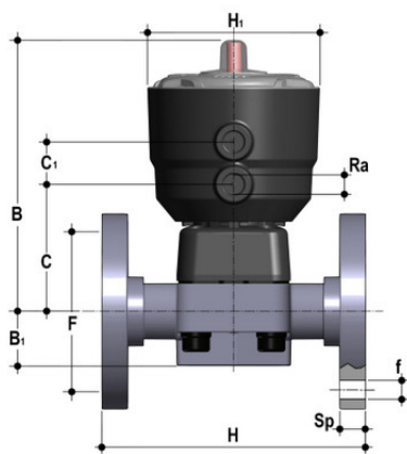
Мембранный клапан DK ХПВХ с пневмоприводом ДвД, PN10, фланцевые окончания d50
