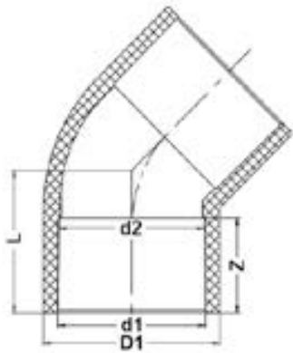
Отвод для раструбной сварки 45° PP-H IPS d25 PN10
