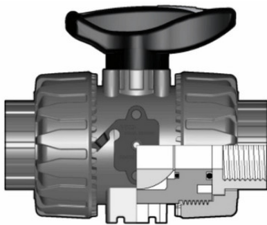
Шаровой кран промышленного применения VKD с резьбовыми окончаниями (уплотнение EPDM) PP-H R3/4" (DN20)
