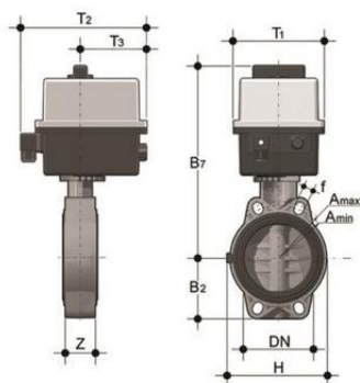
Дисковый затвор общего применения FE ПВХ с эл.приводом 24V AC/DC, EPDM, FIP d140 (DN125)
