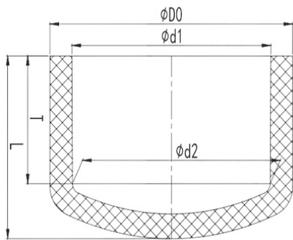
Заглушка клеевая ПВХ IPS d90
