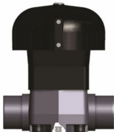
Мембранный клапан VM с пневмоприводом НО с втулочными окончаниями (уплотнение EPDM/мембрана EPDM) PP-H d90 (DN80)
