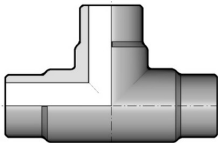
Тройник равнопроходной для стыковой сварки PP-H FIP (PN10) d200 SDR11 PN10
