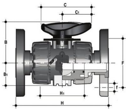
Шаровой кран для регулирования потока VKR с фланцевыми окончаниями (уплотнение FKM) PP-H d32 (DN25)
