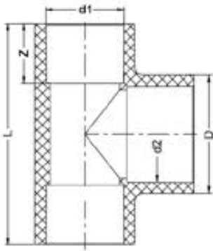
Тройник 90° ХПВХ IPS (Model B) d400 PN10
