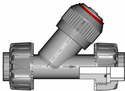
Угловой обратный клапан VRUIV PBX с разборными муфтовыми окончаниями, EPDM, FIP d63 (DN50)
